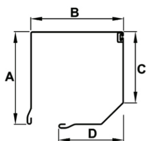
Kaste 45° CLASSIC
